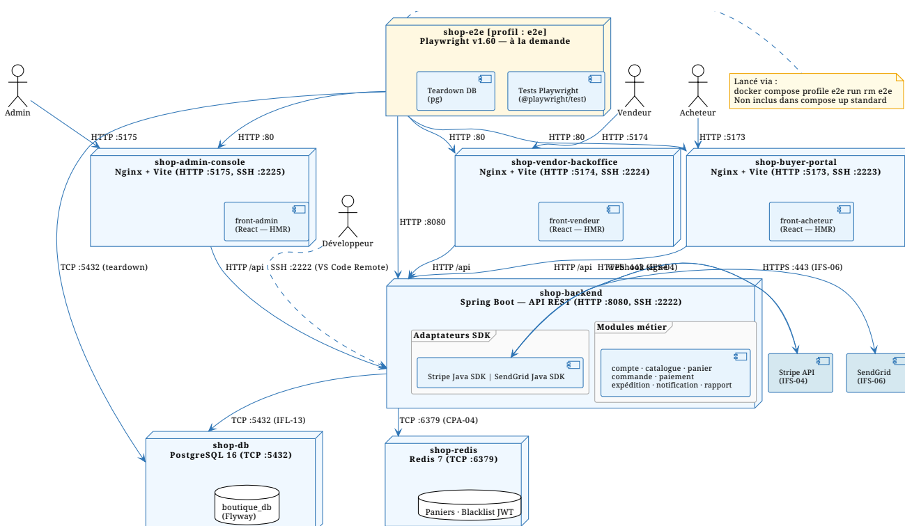
Figure 3. Diagramme de déploiement — environnement de développement
