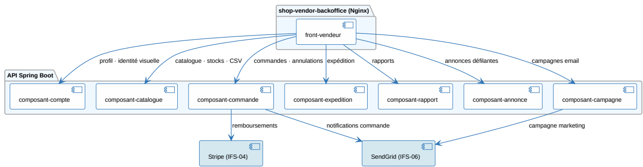
Figure 6. Composants physiques — vue Vendeur
